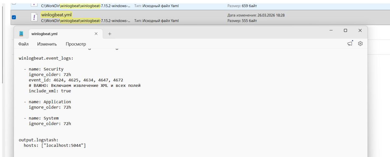
Рисунок 1 – Конфигурация winlogbeat.yml
